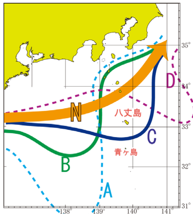
図2 黒潮流型
