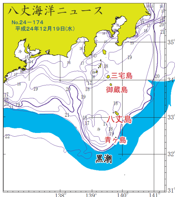
図1 2012年12月19日現在の黒潮流路 (八丈海洋ニュースより)
