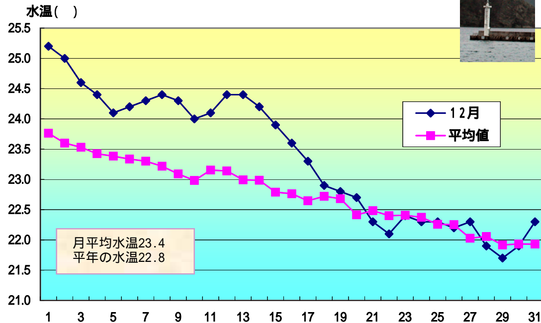
図1 12月の小笠原父島二見湾定地水温記録
