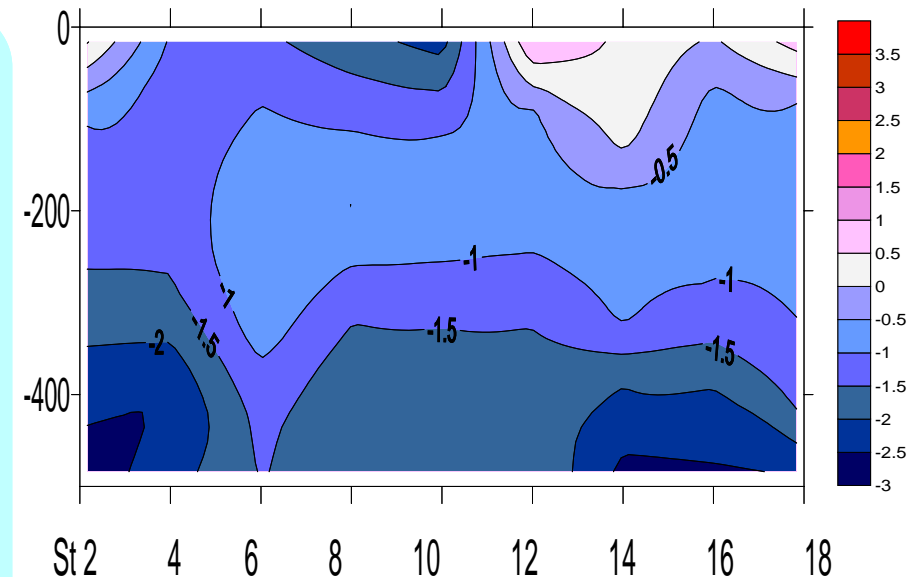
図3 平年差等温線図：縦軸に水深(m)、横軸に小笠原沿岸定線東側のポイント、St2から18までを示した。
