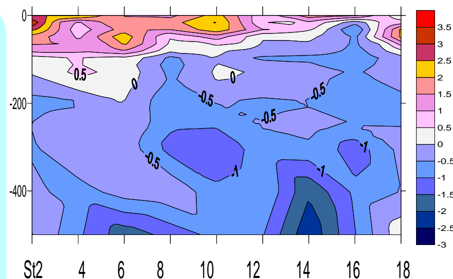
図3 平年差等温線図：縦軸に水深(m)、横軸に小笠原沿岸定線東側のポイント、St2から18までを示した。
