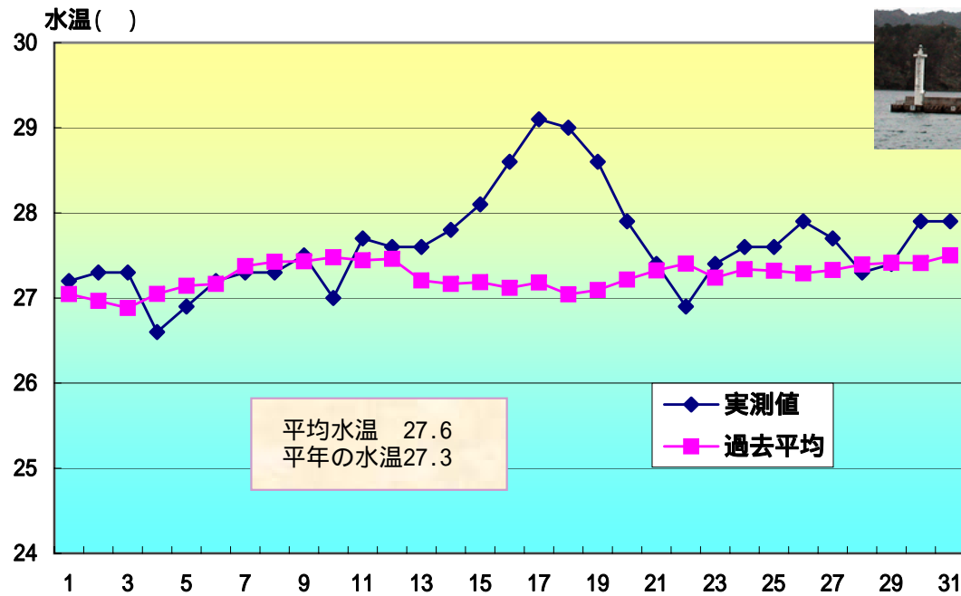
図1 8月の小笠原父島二見湾定地水温記録
