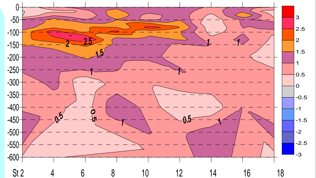
図3 平年差等温線図：縦軸に水深(m)、横軸に小笠原沿岸定線東側のポイント、St2から18までを示した。
