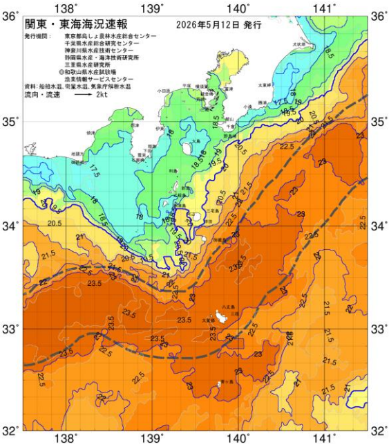
図2 5/12 関東・東海海況速報
