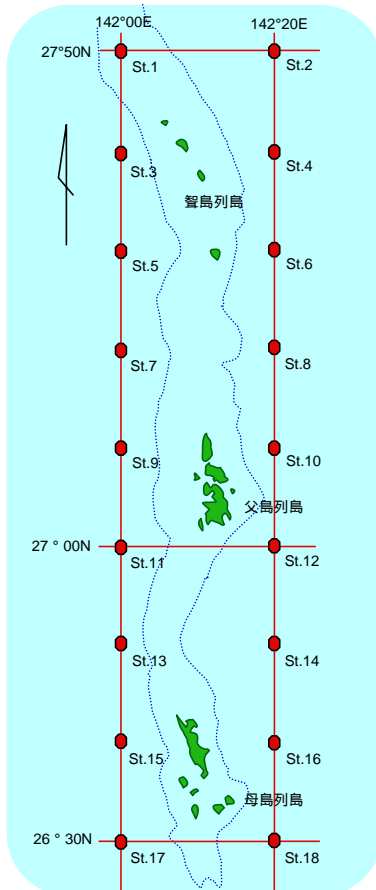
図2 小笠原沿岸観測定点
