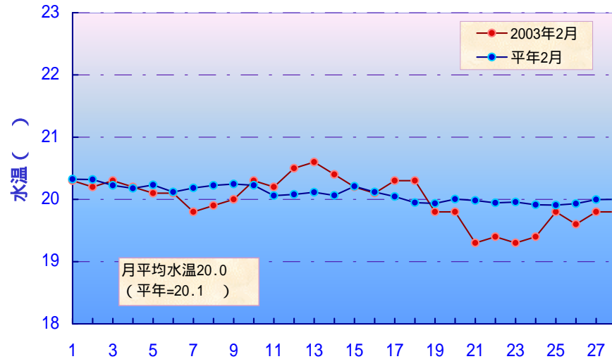
図2 小笠原父島二見湾定地水温記録
