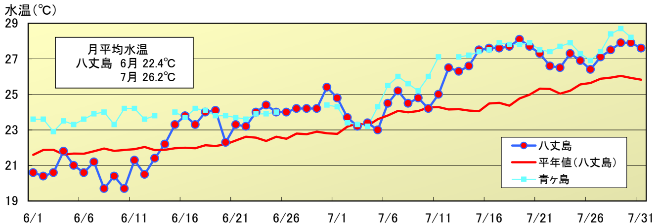
図3 八丈島(神湊港)における6-7月の定地水温観測結果
