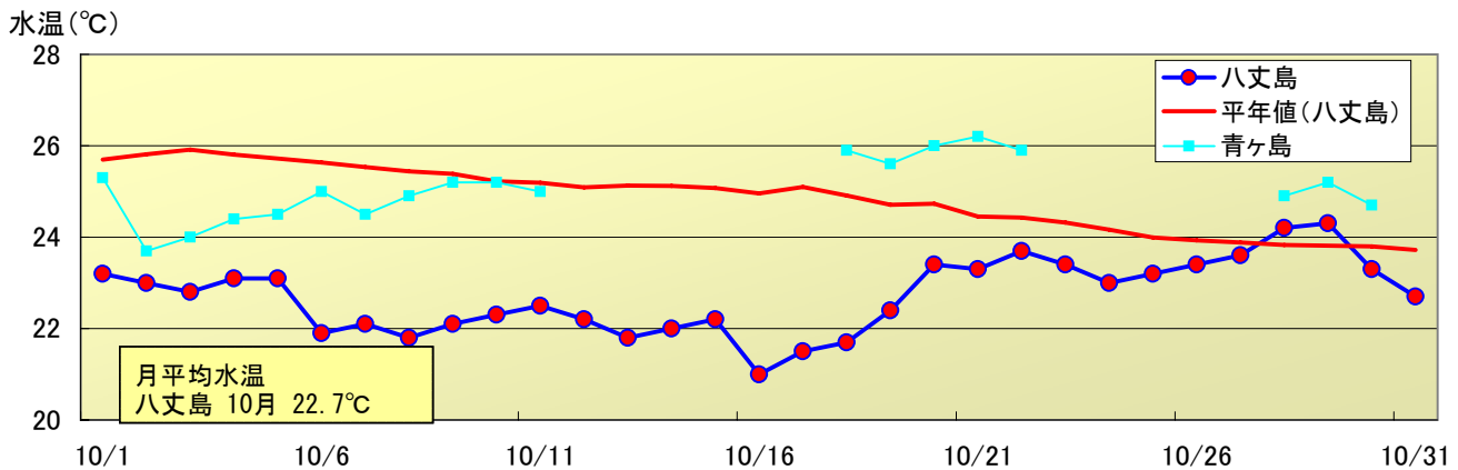
図3 八丈島(神湊港)における10月の定地水温観測結果
