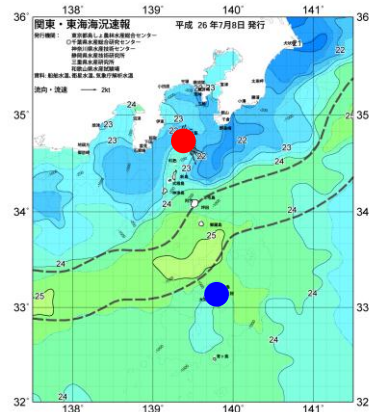
図2 7/8の海況
