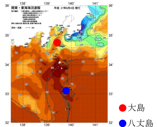
図2 8/4の海況図
