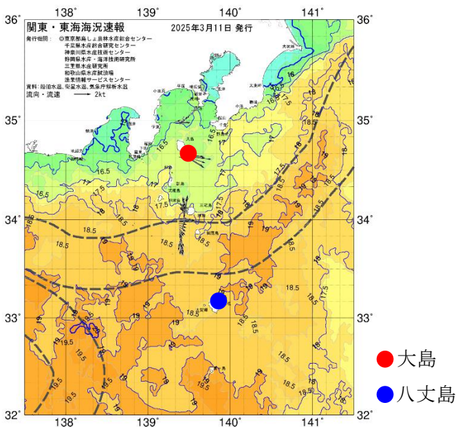
図2 3/11の海況図
