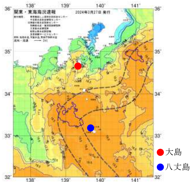
図2 3/27の海況図
