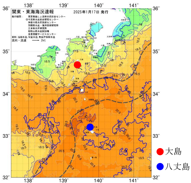
図2 1/17 の海況図
