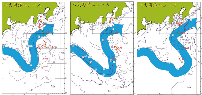
図1 2025年6月の黒潮流路
