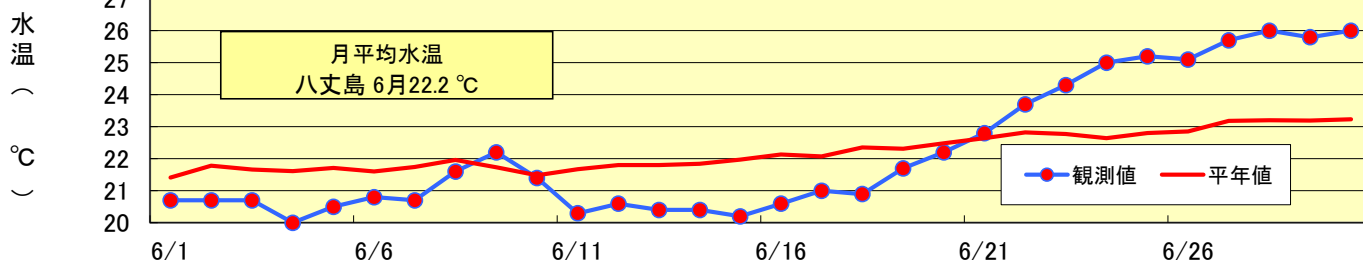
図3 八丈島(神湊港)における6月の定地水温観測結果
