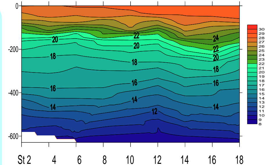
図3 等温線図：縦軸に水深、横軸に小笠原沿岸定線東側のポイント、St2から18までを示した。
