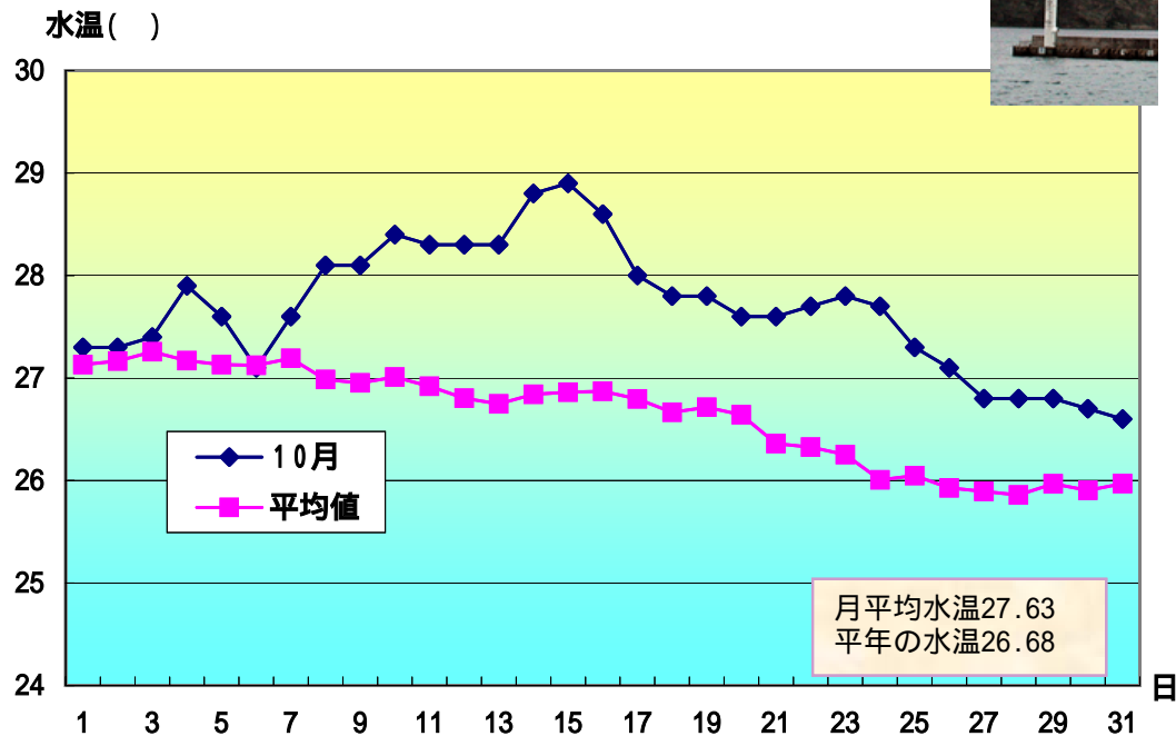
図1 10月の小笠原父島二見湾定地水温記録
