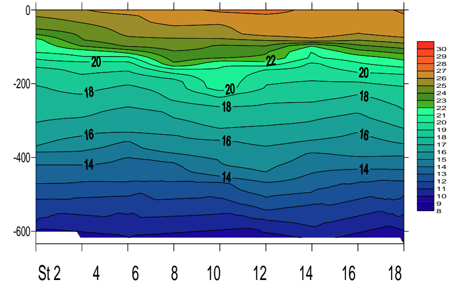
図3 等温線図：縦軸に水深、横軸に小笠原沿岸定線東側のポイント、St2から18までを示した。
